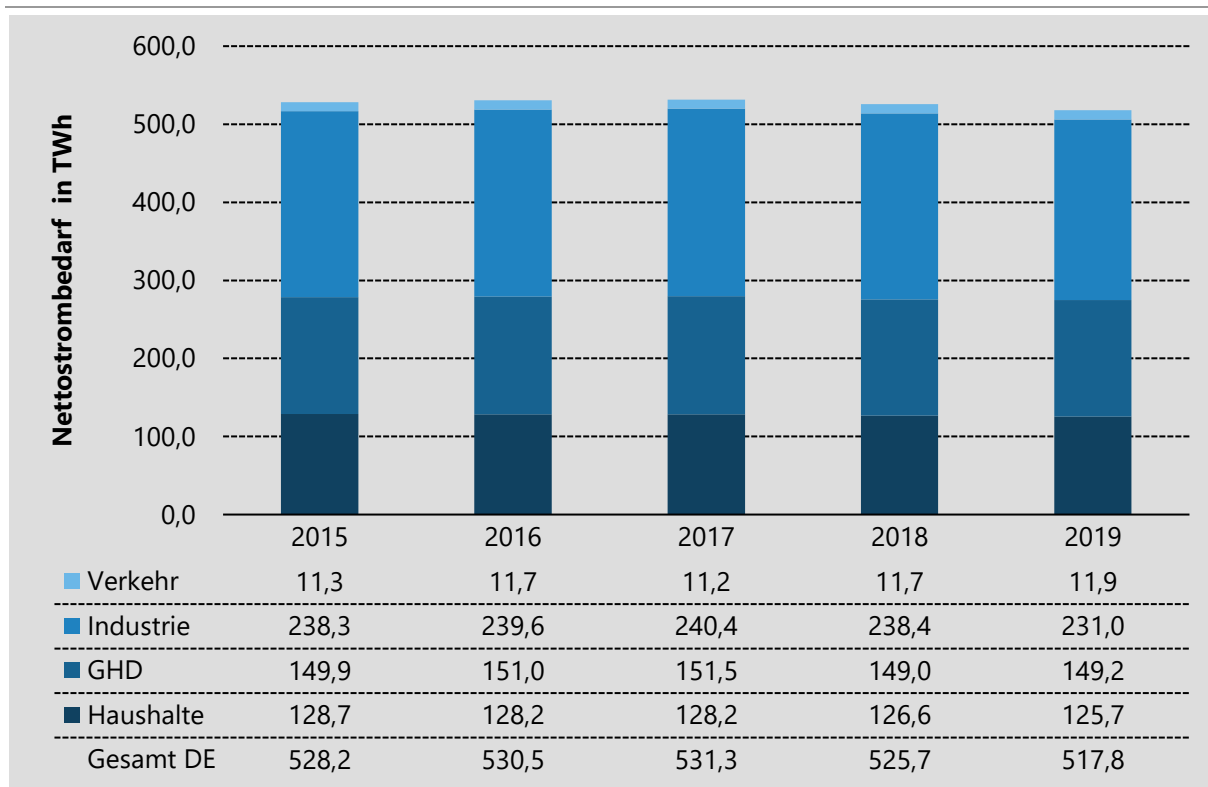
Abbildung 2: Historie des Nettostrombedarfs für die Jahre 2015 bis 2019 (nicht temperaturbereinigt)
