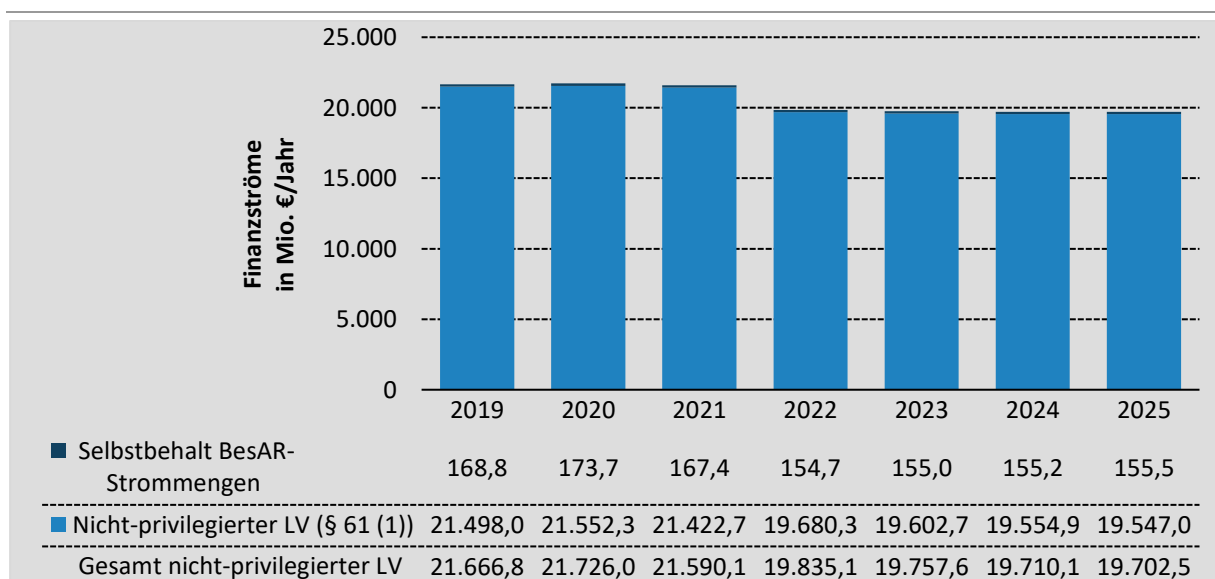
Abbildung 17: Entwicklung der Finanzströme des nicht-privilegierten Letztverbrauchs für die Jahre 2019 bis 2025
