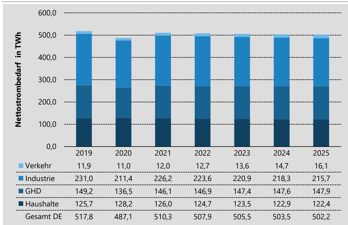
Abbildung 9: Entwicklung des Nettostrombedarfs im Referenzszenario
