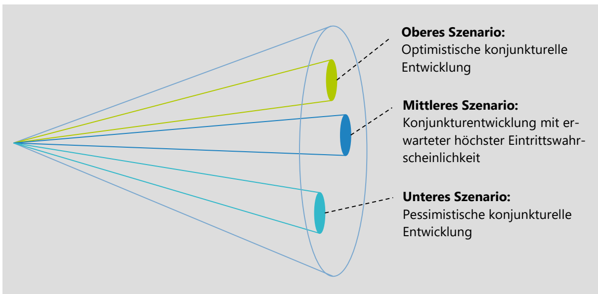
Abbildung 6: Szenariotrichter
