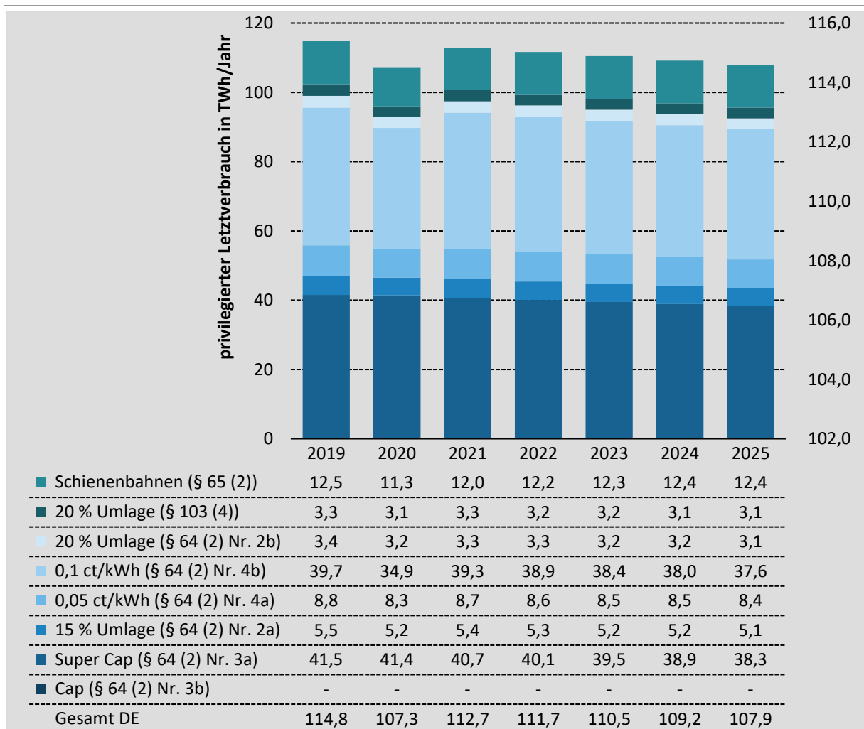
Abbildung 14: Entwicklung der Strommengen des privilegierten Letztverbrauchs nach Begrenzungstatbeständen für die Jahre 2019 bis 2025
