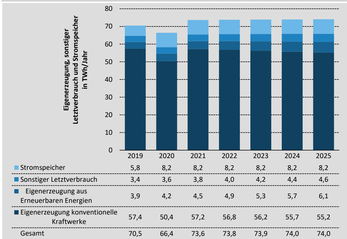
Abbildung 11: Entwicklung der Eigenerzeugung, des sonstigen Letztverbrauchs sowie Lieferungen an Speicher im Referenzszenario für die Jahre 2019 bis 2025
