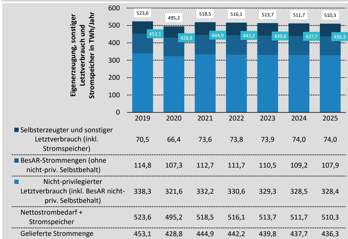
Abbildung 10: Entwicklung des nicht-privilegierten, privilegierten sowie selbsterzeugten und sonstigen Letztverbrauch für die Jahre 2019 bis 2025
