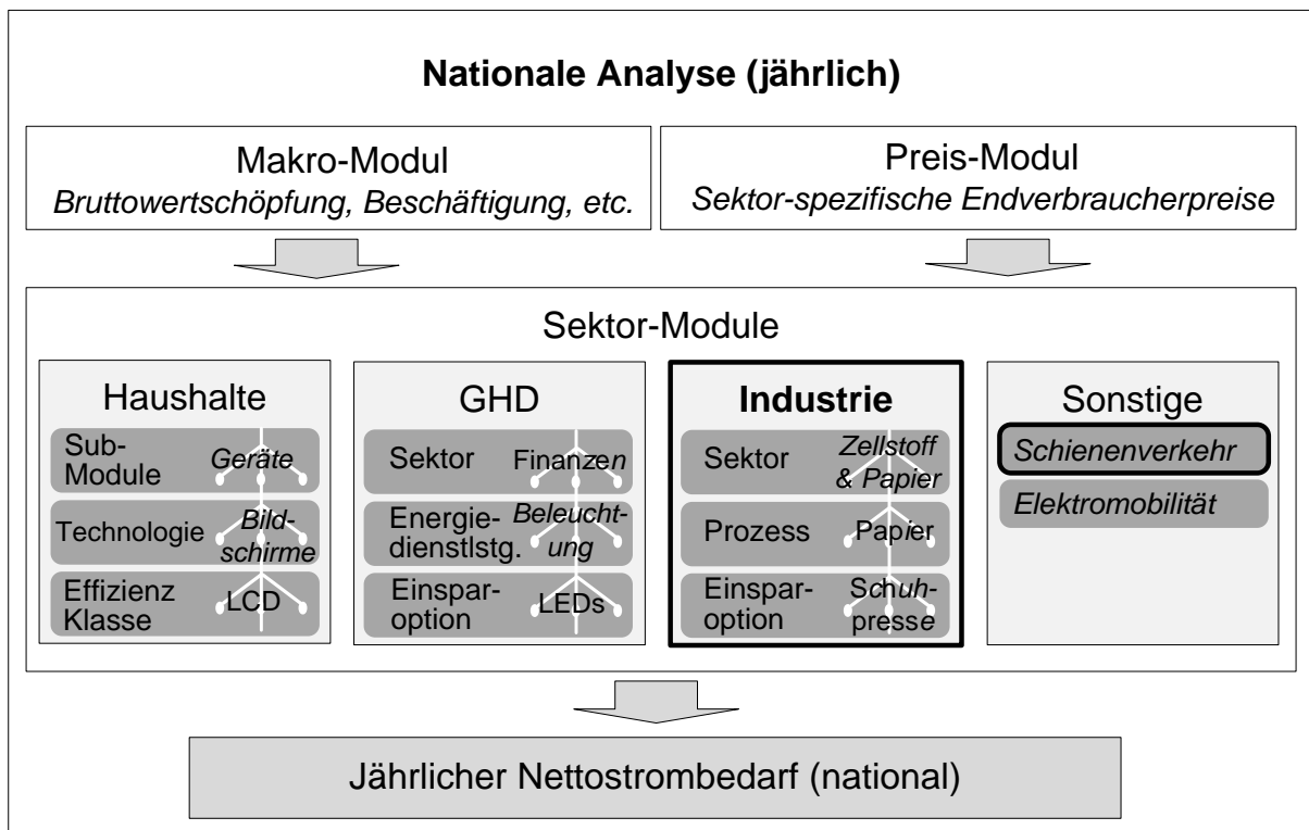
Abbildung 1: Schematische Darstellung der nationalen Analyse (jährlich)
