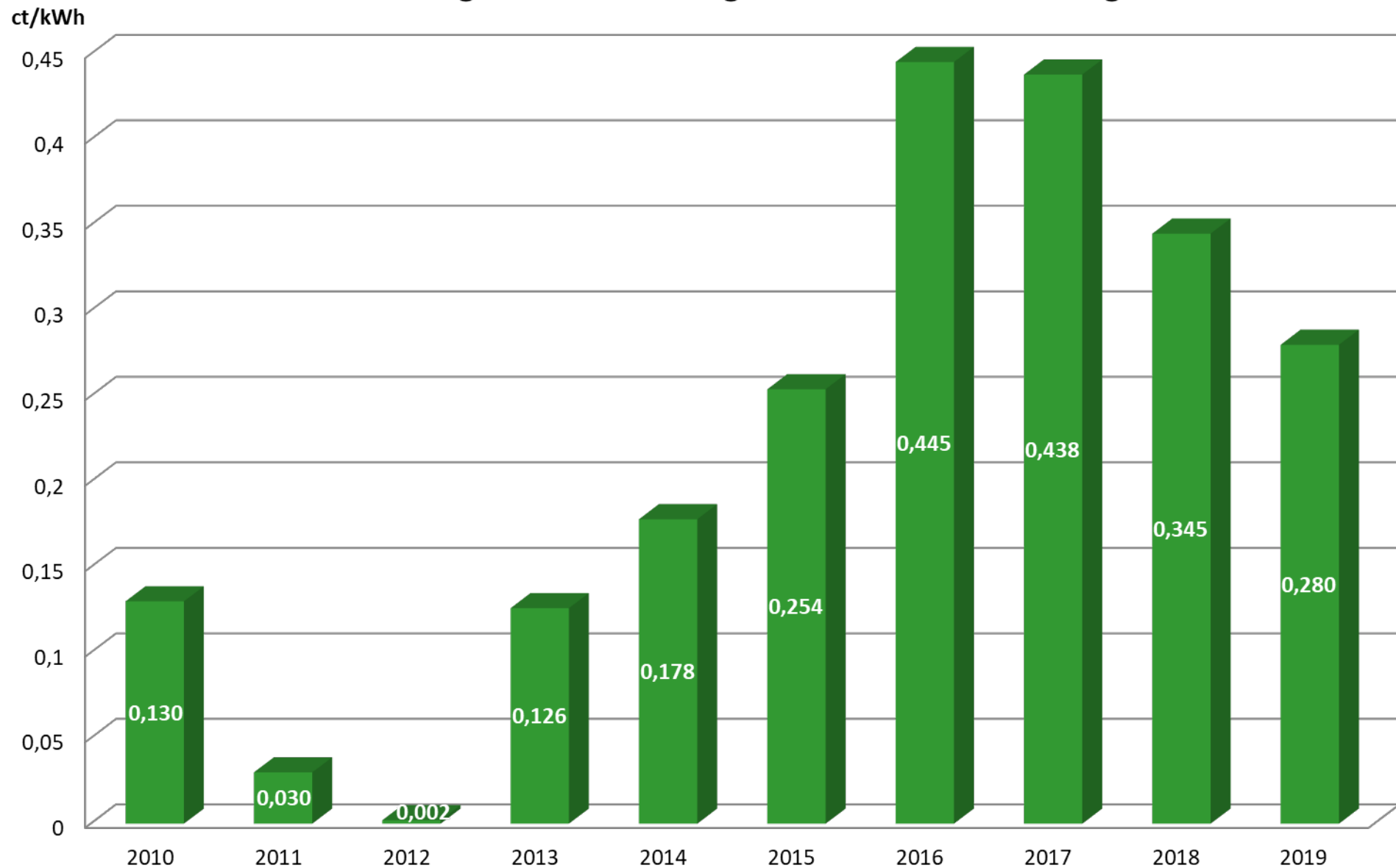
Entwicklung der KWKG-Umlage bzw. des KWK-Aufschlags
