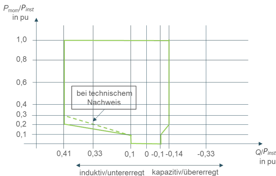
Abbildung 10 Anforderung an die Blindleistungsbereitstellung von Elektrolyseanlagen im Teillastbetrieb im Verbrauchszählpfeilsystem
