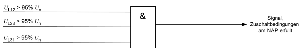
Abbildung 6: Bildung des Signals für die Zuschaltbedingungen am Netzanschlusspunkt.
