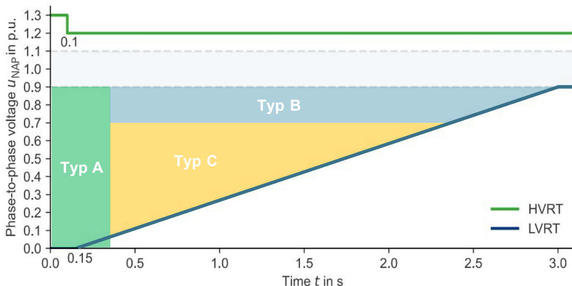
Abbildung 3 Bereiche der Ausnahmeregelung an die FRT-Fähigkeit und die Wiederkehr der Wirkleistungsaufnahme in Abhängigkeit von der Dauer und Tiefe eines Spannungseinbruchs während eines Netzfehlers.
