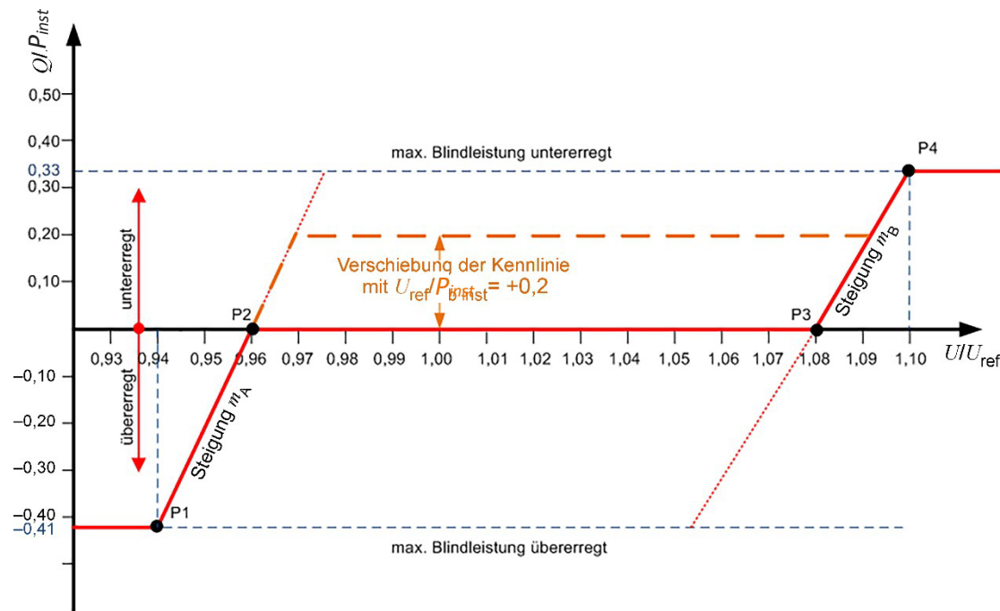
Abbildung 12: Beispiel für eine Q-Vorgabe
