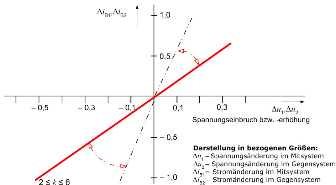
Abbildung 8: Prinzip der Spannungsstützung bei Netzfehlern
