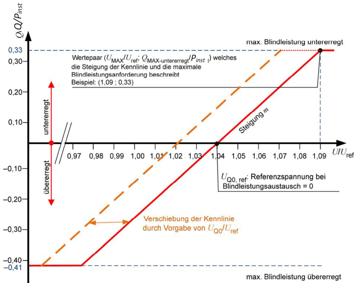
Abbildung 11 Beispiel für eine Q(U)-Kennlinie
