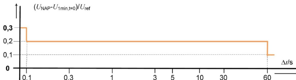
Abbildung 1: Grenzkurve für relative Spannungserhöhungen
