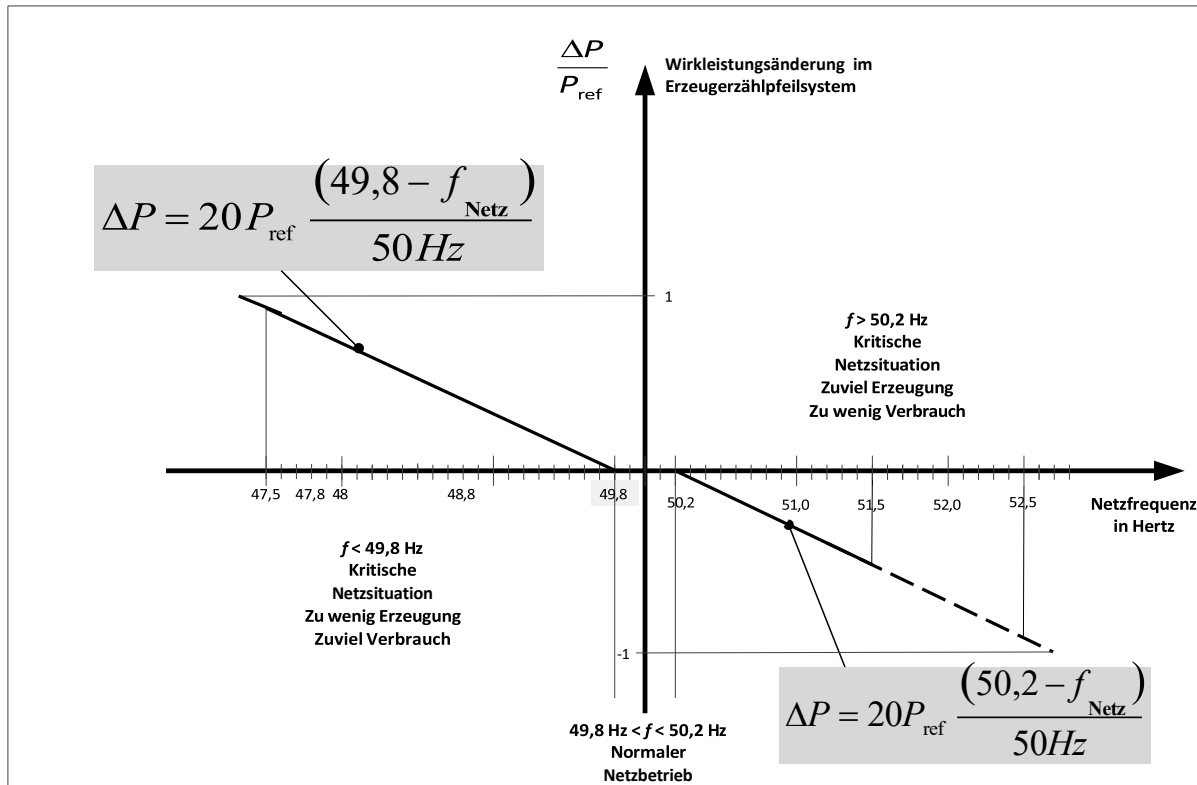
Abbildung 5: Wirkleistungsanpassung stufenlos steuerbarer Elektrolyseanlagen bei Über- und Unterfrequenz mit einer Statik von 5 % und Frequenzgrenzwerten von 49,8 Hz und 50,2 Hz für den Beginn der Wirkleistungsanpassung
