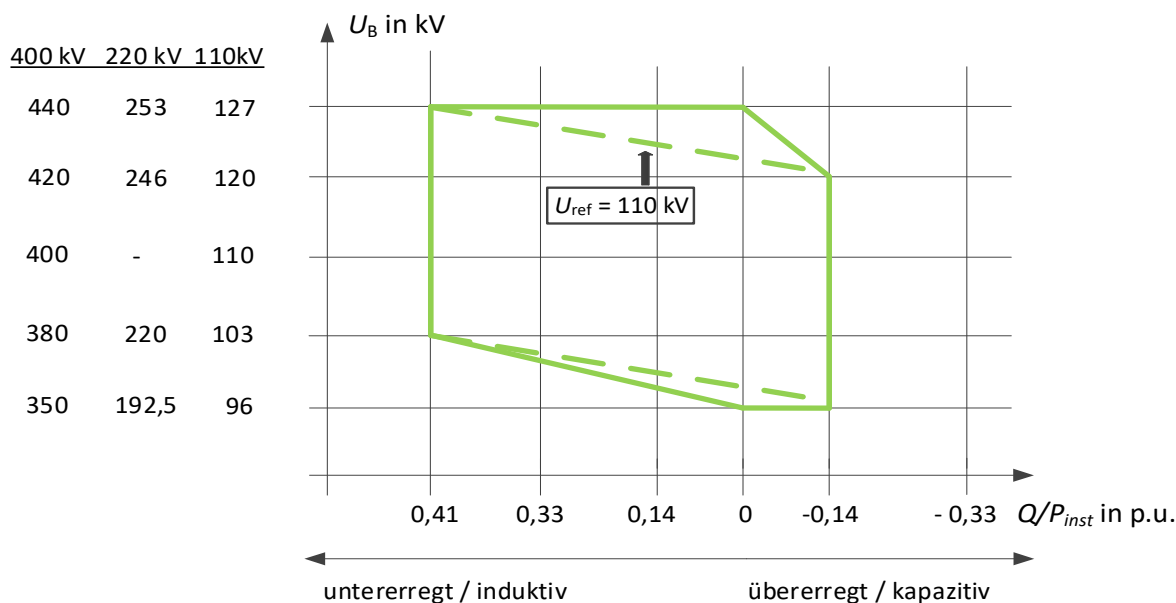
Abbildung 9 Anforderungen zu Blindleistungsabgabe bzw. -bezug am Netzanschlusspunkt im Verbraucherschlupfsystem
