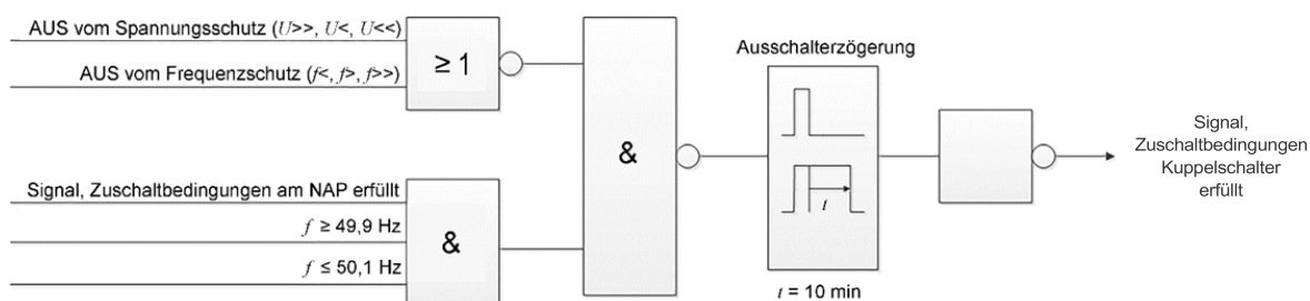
Abbildung 7: Funktionsschema der automatischen Zuschaltung eines Kuppelschalters.
